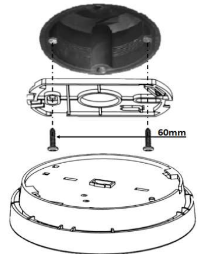
Geeignet zur Montage auf Standard UP-Dosen Lochabstand 60mm
