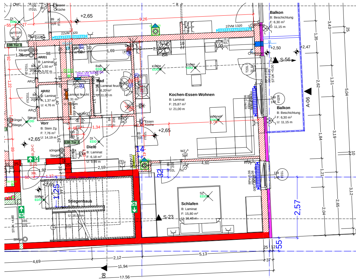
1.Stock; 2B; 1:100; 01.09.2015; Vorbehaltlich technischer Änderungen
